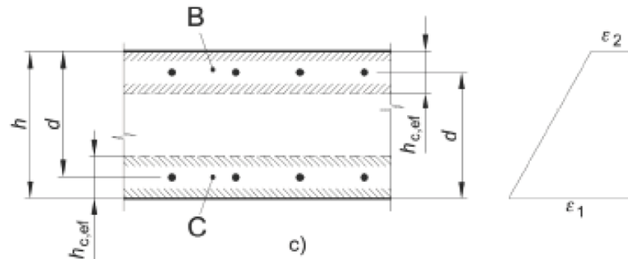
Figura C4.1.10- Area tesa efficace. Casi tipici
