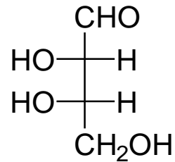
L-ERITROSIO
