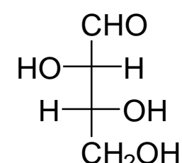
D-TREOSIO
