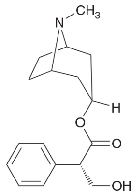
atropina
