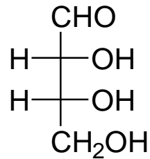
D-ERITROSIO
