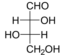
L-TREOSIO
