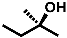
2-butanolo
