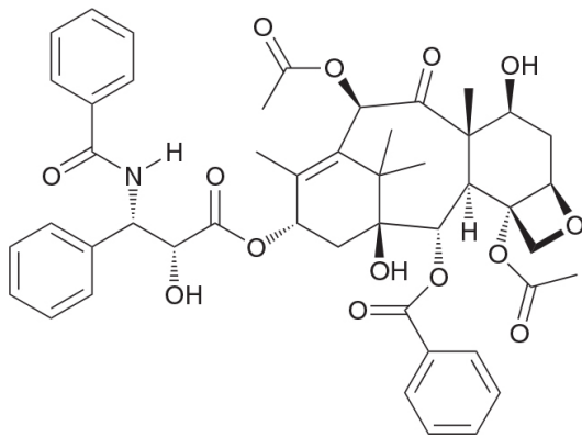
Taxol
