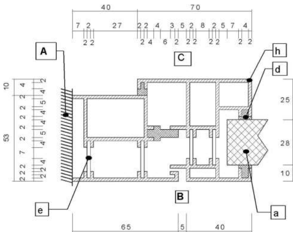
Figura 136: Infisso in alluminio a taglio termico
