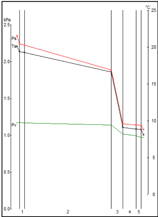
Figura 281: Verifica Glaser per il solaio
