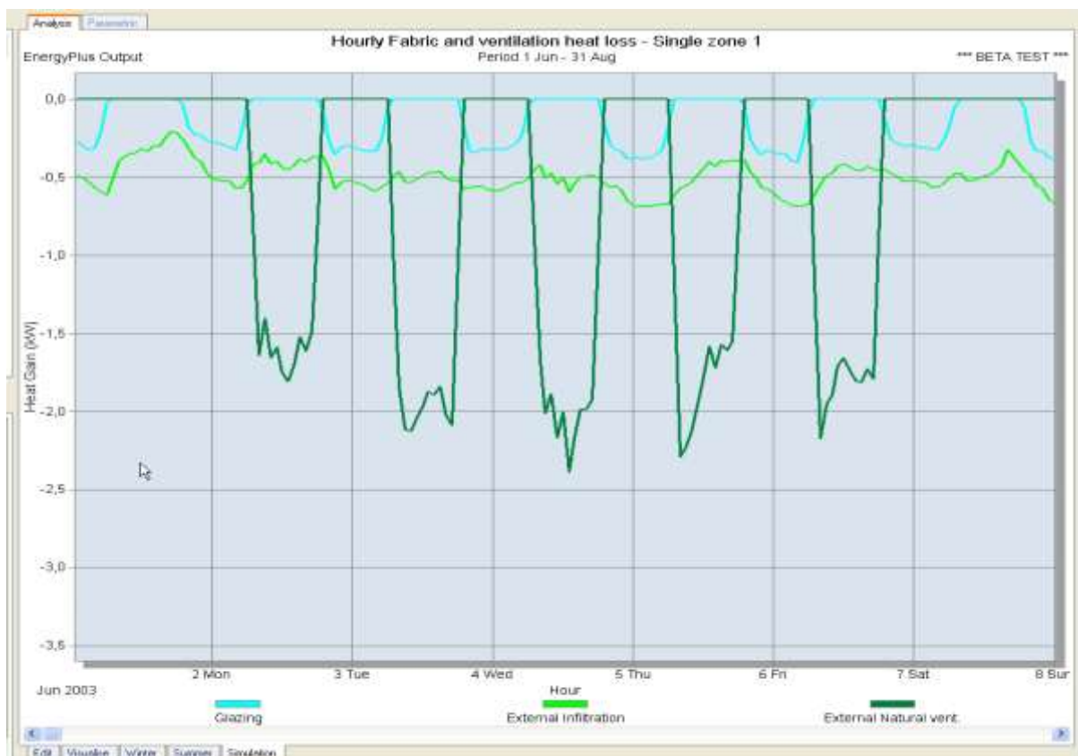
Figura 220: Visualizzazione delle perdite per ventilazione
