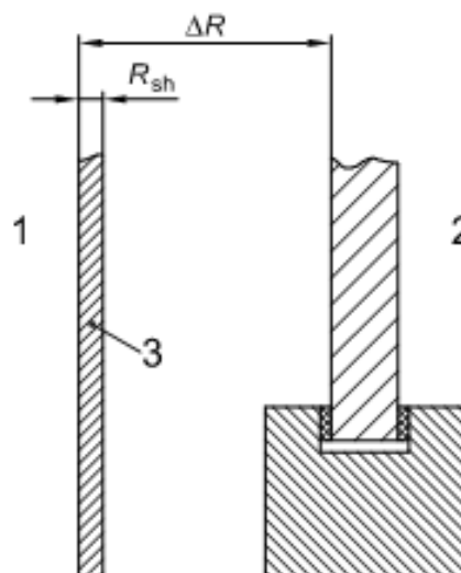
Figura 131: Finestra con chiusura esterna
