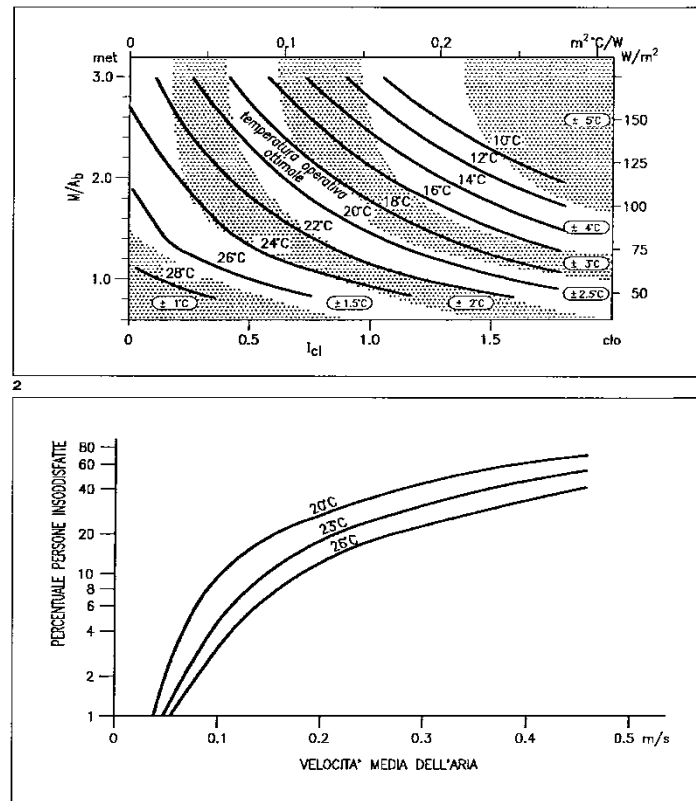
Figura 62: Condizioni di benessere ( M/A_b , t_{cl} ) e della PPD al variare della velocità media dell'aria.
