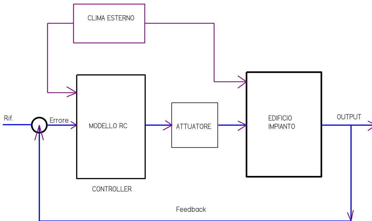
Figura 251: Sistema di controllo dell'edificio con l'utilizzo del modello ridotto
