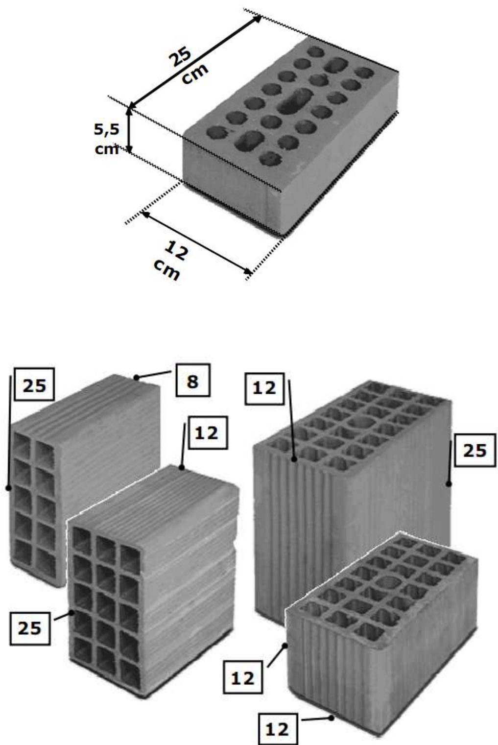
Figura 87: Esempio di matton1 forat1
