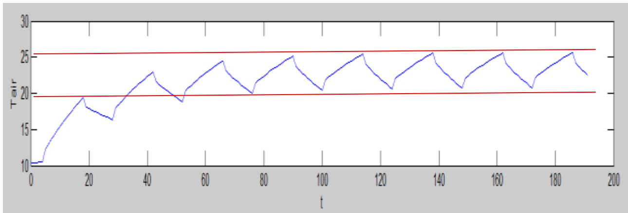
Figura 243: Transitorio termico per 7 giorni con 2C – particolare di T_{air}
