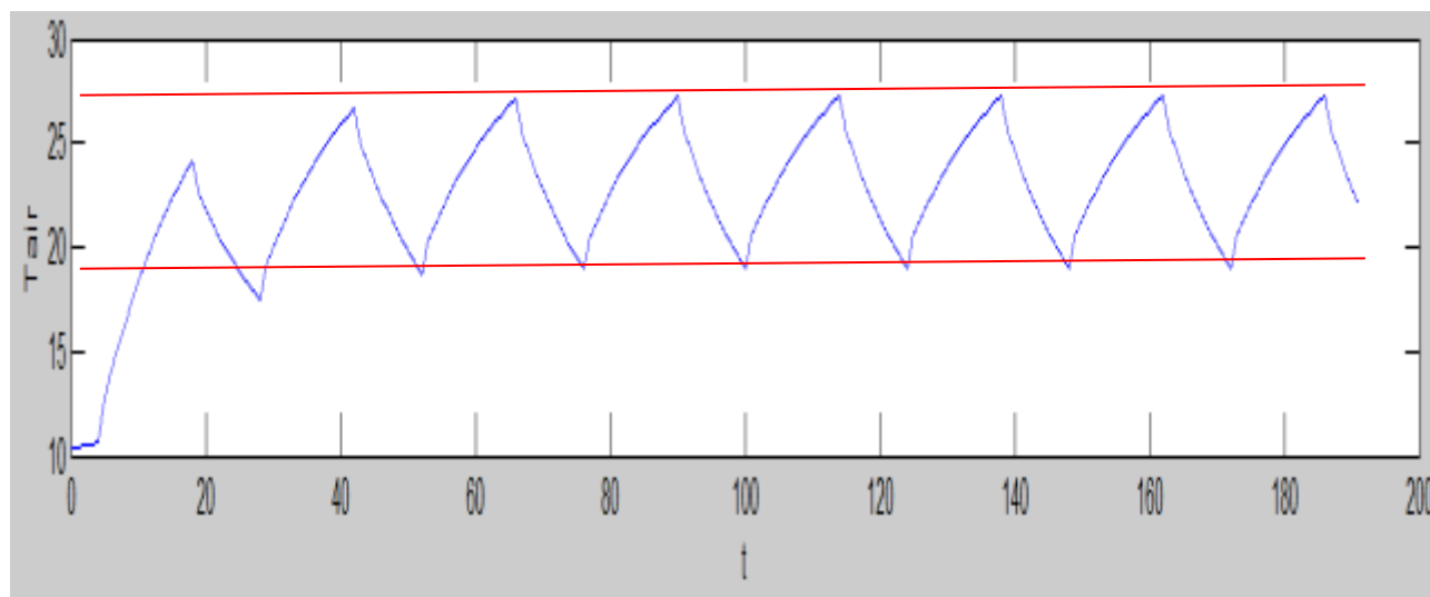
Figura 240: Transitorio termico per 7 giorni – particolare della T_{air}
