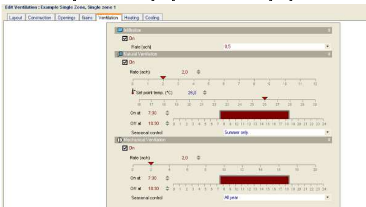
Figura 205: Selezione del tipo di ventilazione
