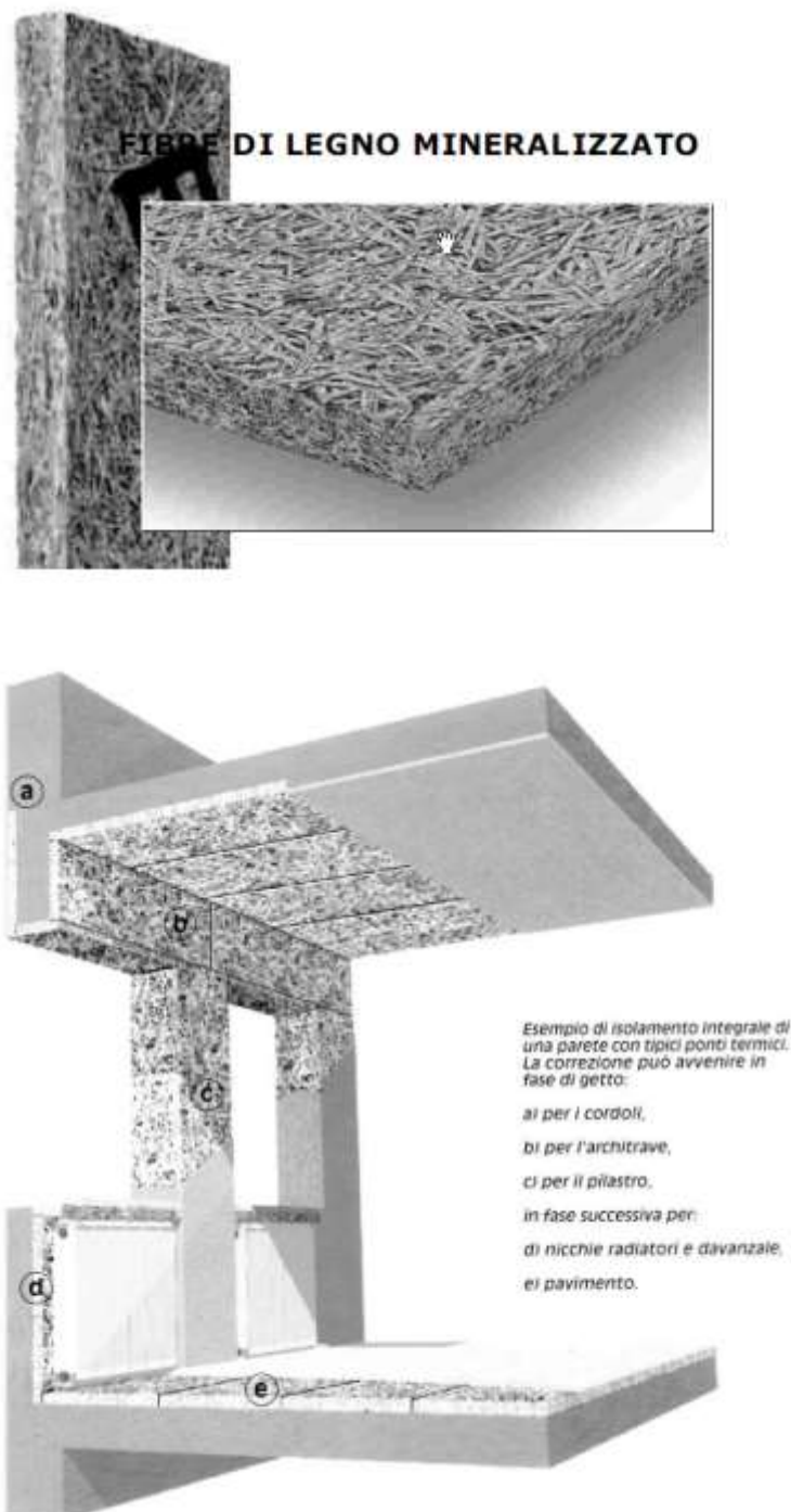
Figura 92: Pannello di legno mineralizzato
