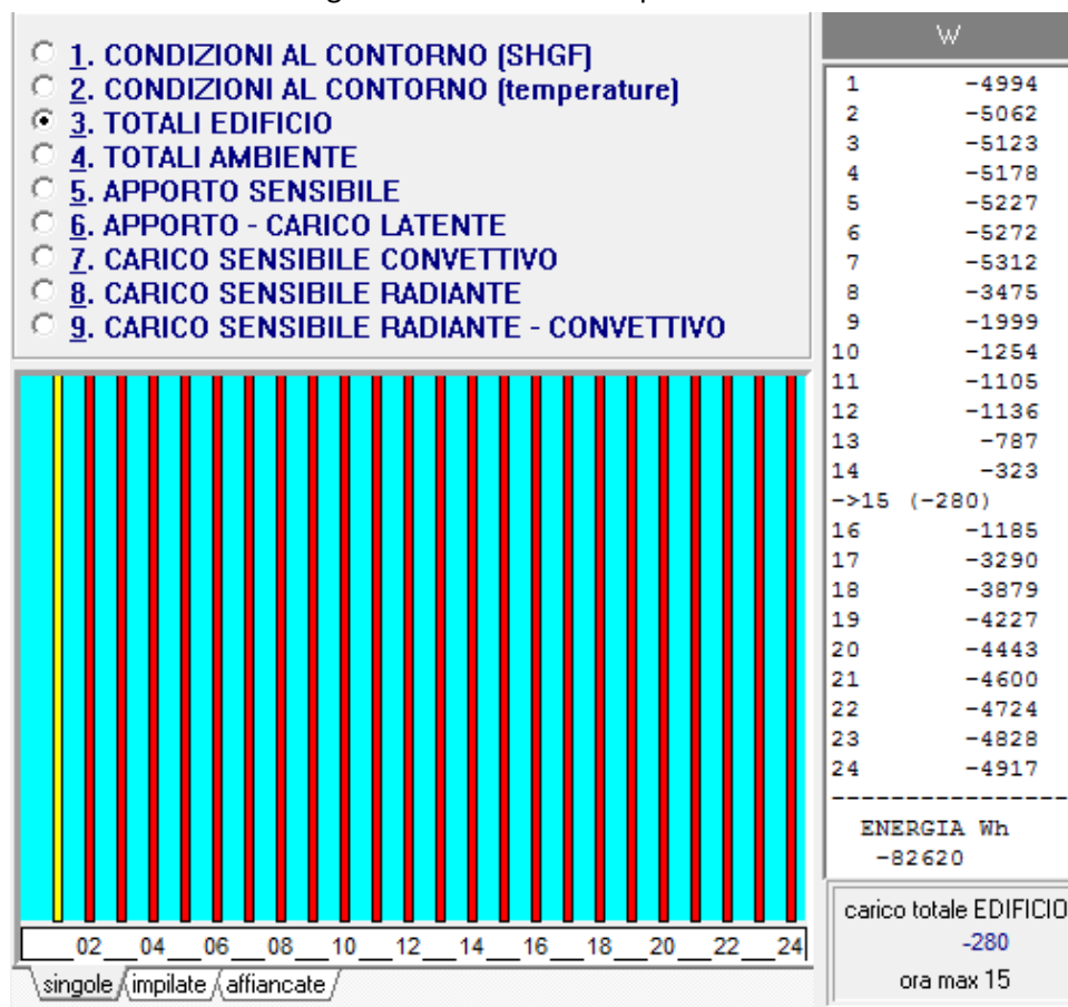
Figura 264: Carico dinamico a gennaio
