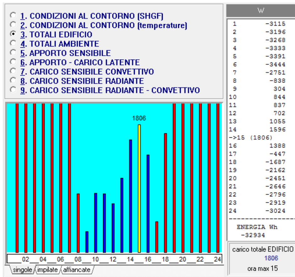
Figura 265: Carico dinamico a febbraio
