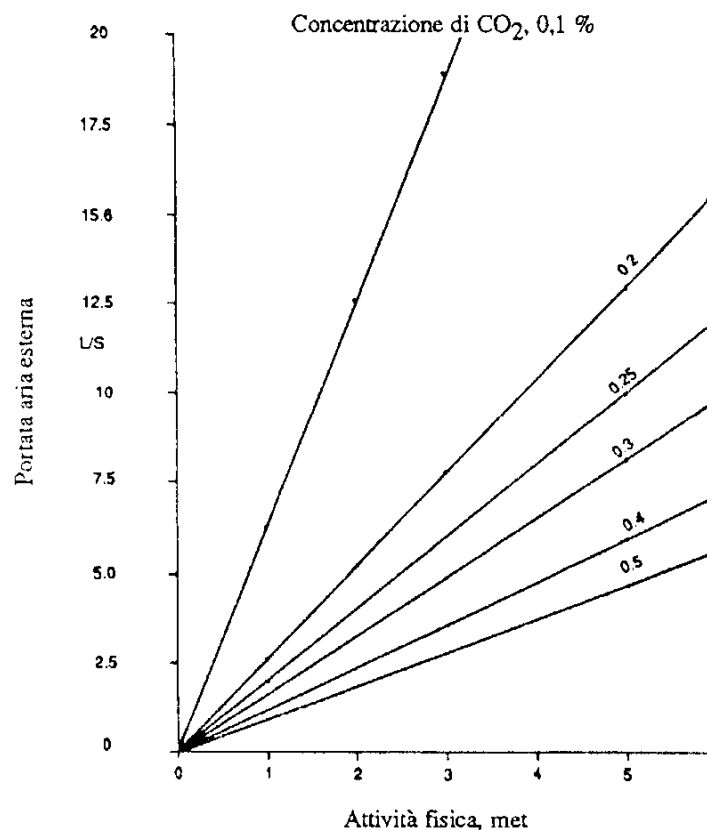
Figura 71: Portata di aria esterna al variare dell'attività fisica e della % di \text{CO}_2
