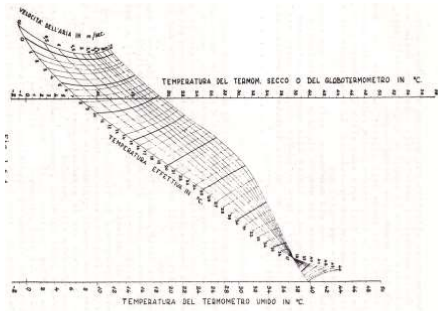
Figura 57: Temperatura effettiva per persone vestite
