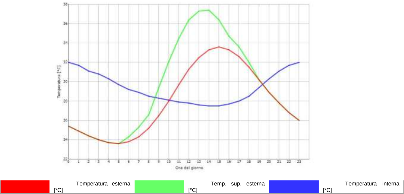
Figura 182: Diagramma di sfasamento dell'onda termica
