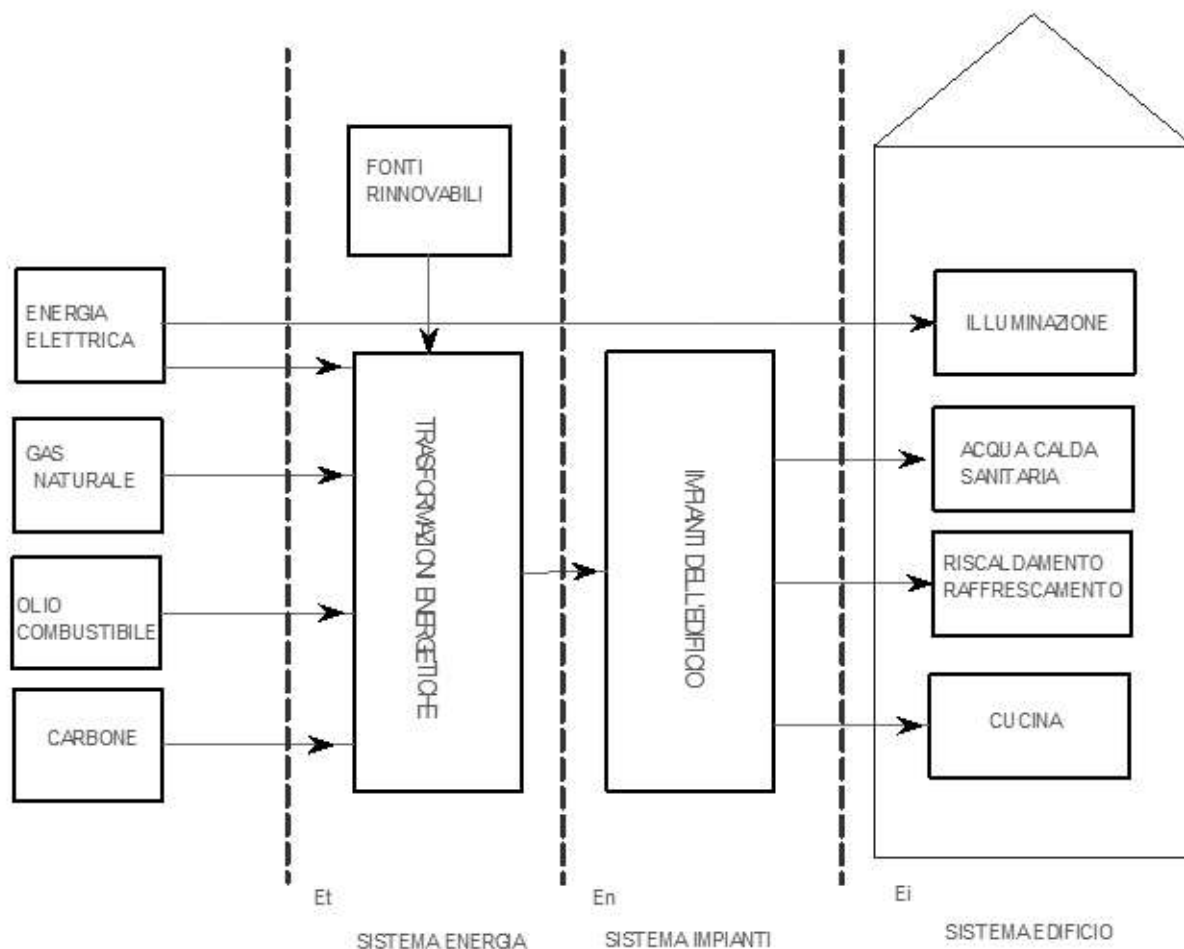
Figura 53: Sistema edificio-impianto
