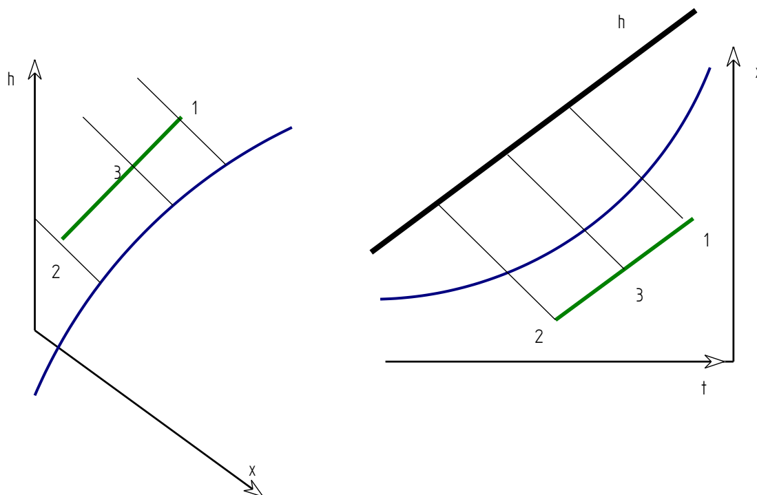
Figura 18: Rappresentazione della miscelazione adiabatica di due correnti d'aria umida
