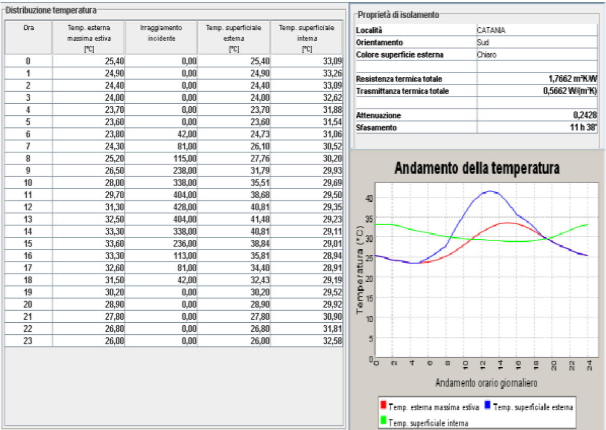
Figura 169: Parete di Figura 166 ma esposta a sud
