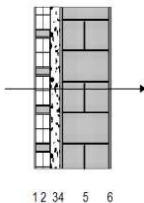
Figura 276: Stratigrafia di una parete composta
