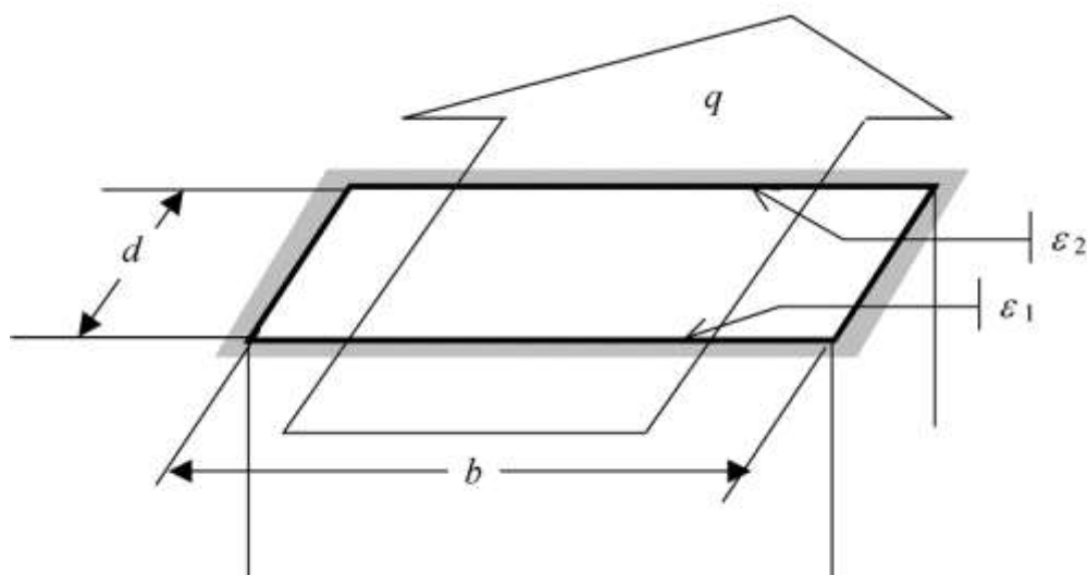
Figura 135: Cavità rettangolare e direzione del flusso
