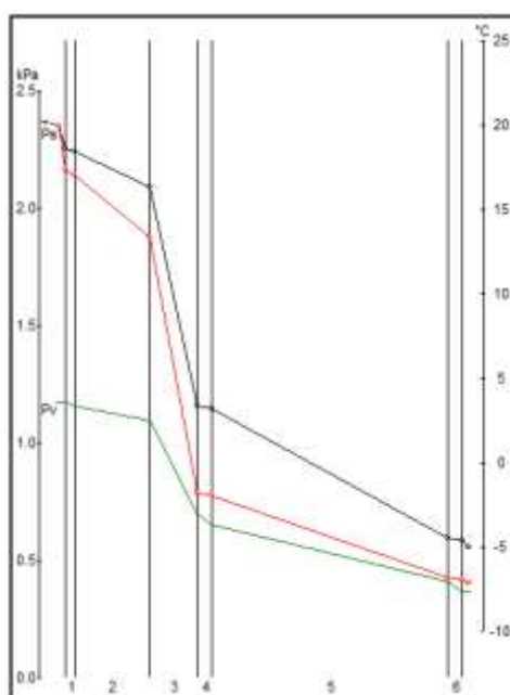
Figura 276: Stratigrafia di una parete composta
