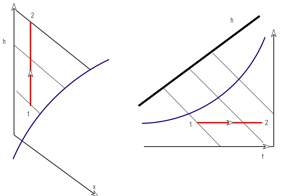
Figura 19: Rappresentazione del riscaldamento dell'aria umida.
