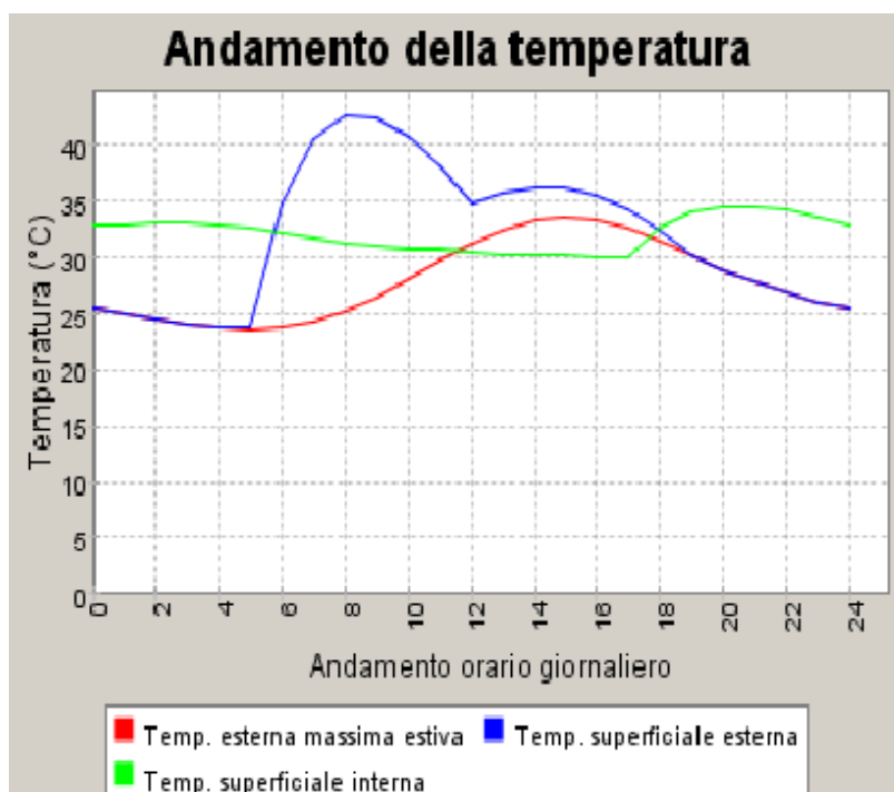
Figura 168: Andamento delle temperature superficiali per la parete di Figura 166 esposta ad est
