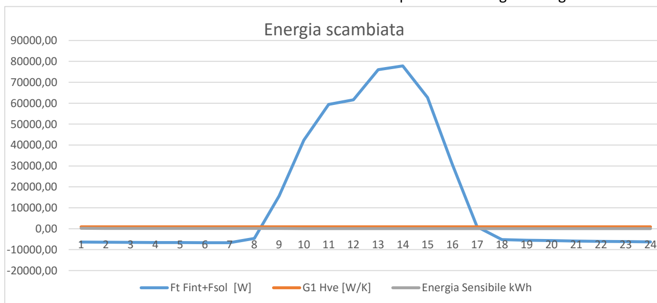
Figura 257: Flussi termici calcolati per l'edificio esempio
