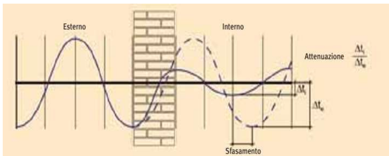
Figura 150: Azione di una parete sull'onda termica
