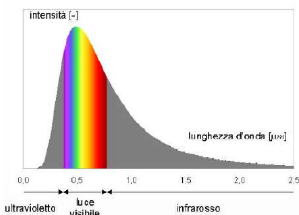
Figura 164: Spettro solare ideale
