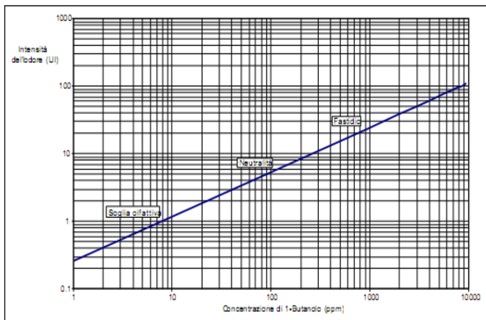
Figura 79: Scala di riferimento del Butanolo
