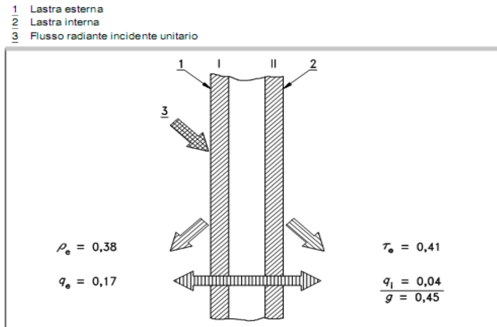
Figura 138: Ripartizione del flusso solare incidente
