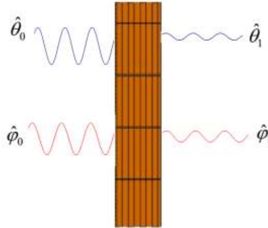
Figura 178: Rappresentazione del quadripolo equivalente della parete
