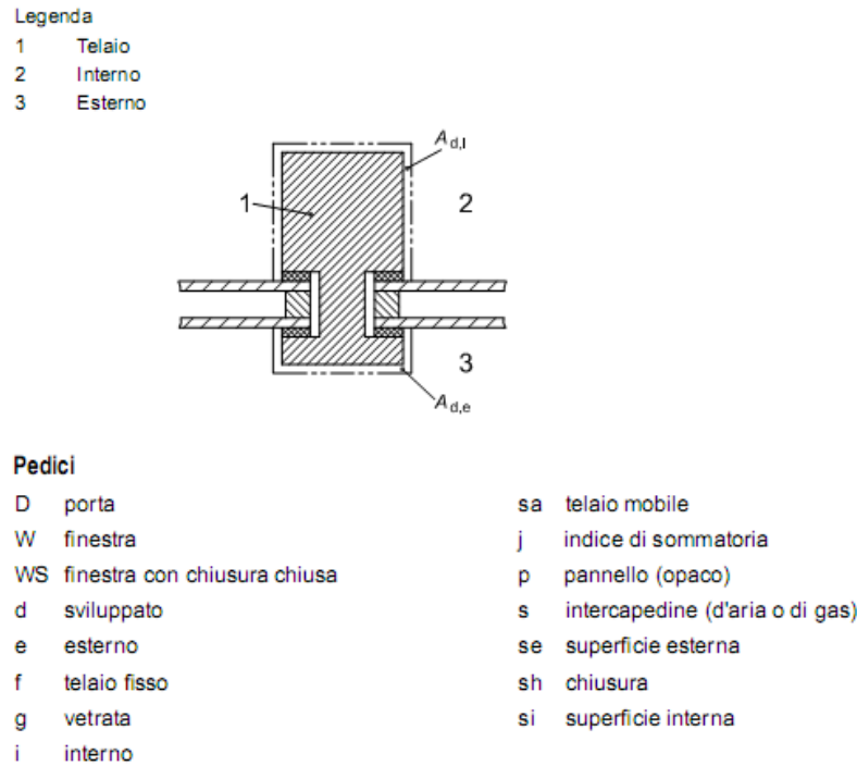
Figura 124: Sviluppo dell'area interna ed esterna
