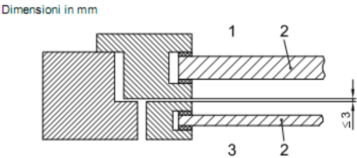
Figura 129: Schematizzazione di finestre accoppiate
