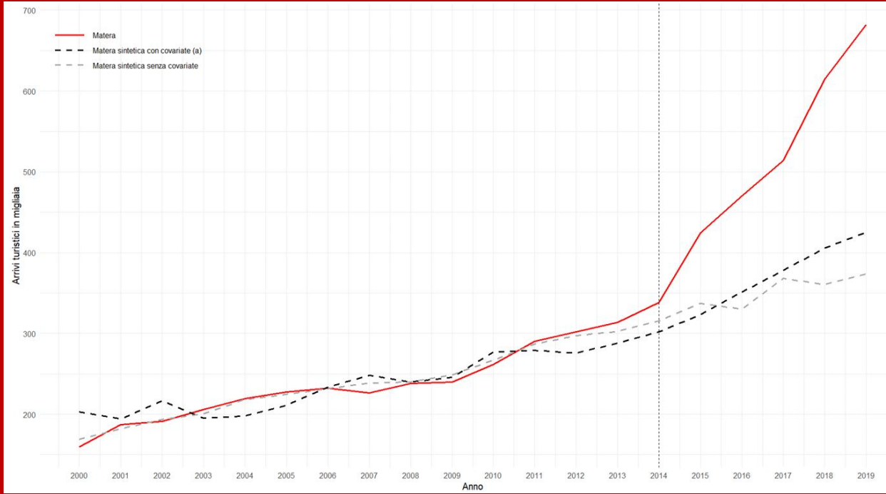
«Covariate a»
