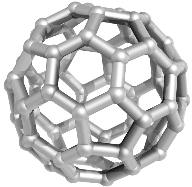
icosaedro troncato (fullerene, 1985)
